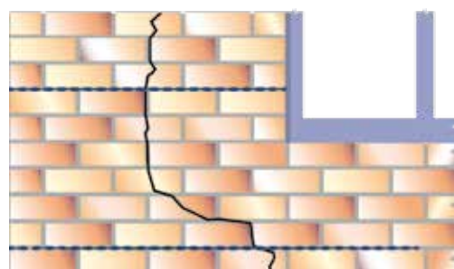
Popravka pukotina u blizini uglova i otvora (videti prospekt o popravci pukotina)
