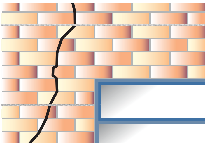
Réparation d'une fissure dans un mur en brique classique au moyen de la barre SureTwist.
